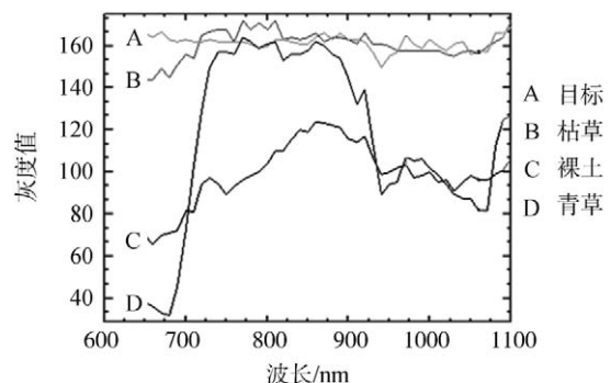
图6 高光谱遥感影像目标探测实验中主要地物的光谱曲线
