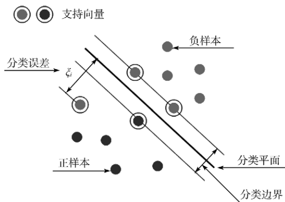
图2 SVM 分类器使得正样本与负样本之间的距离最大
